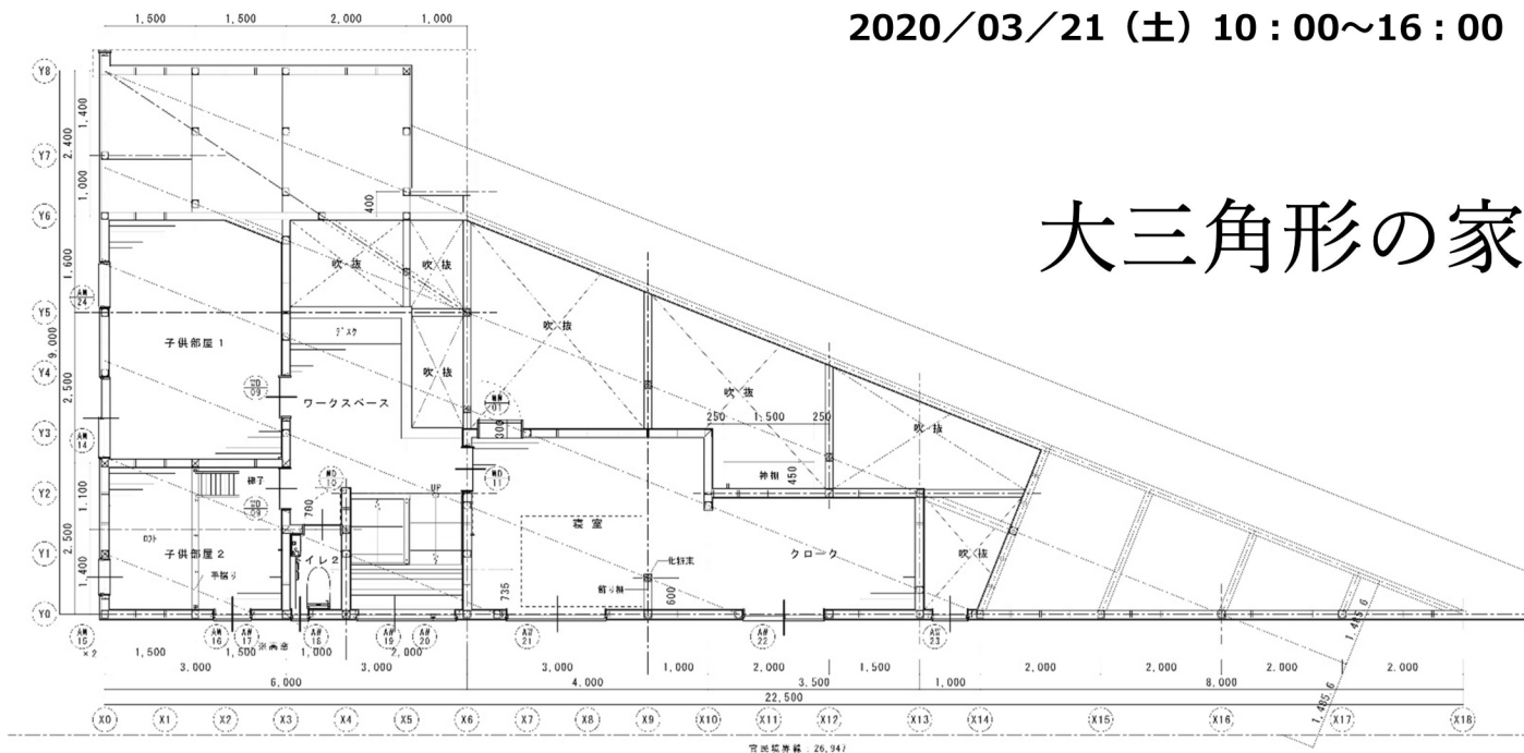
2階平面詳細図
