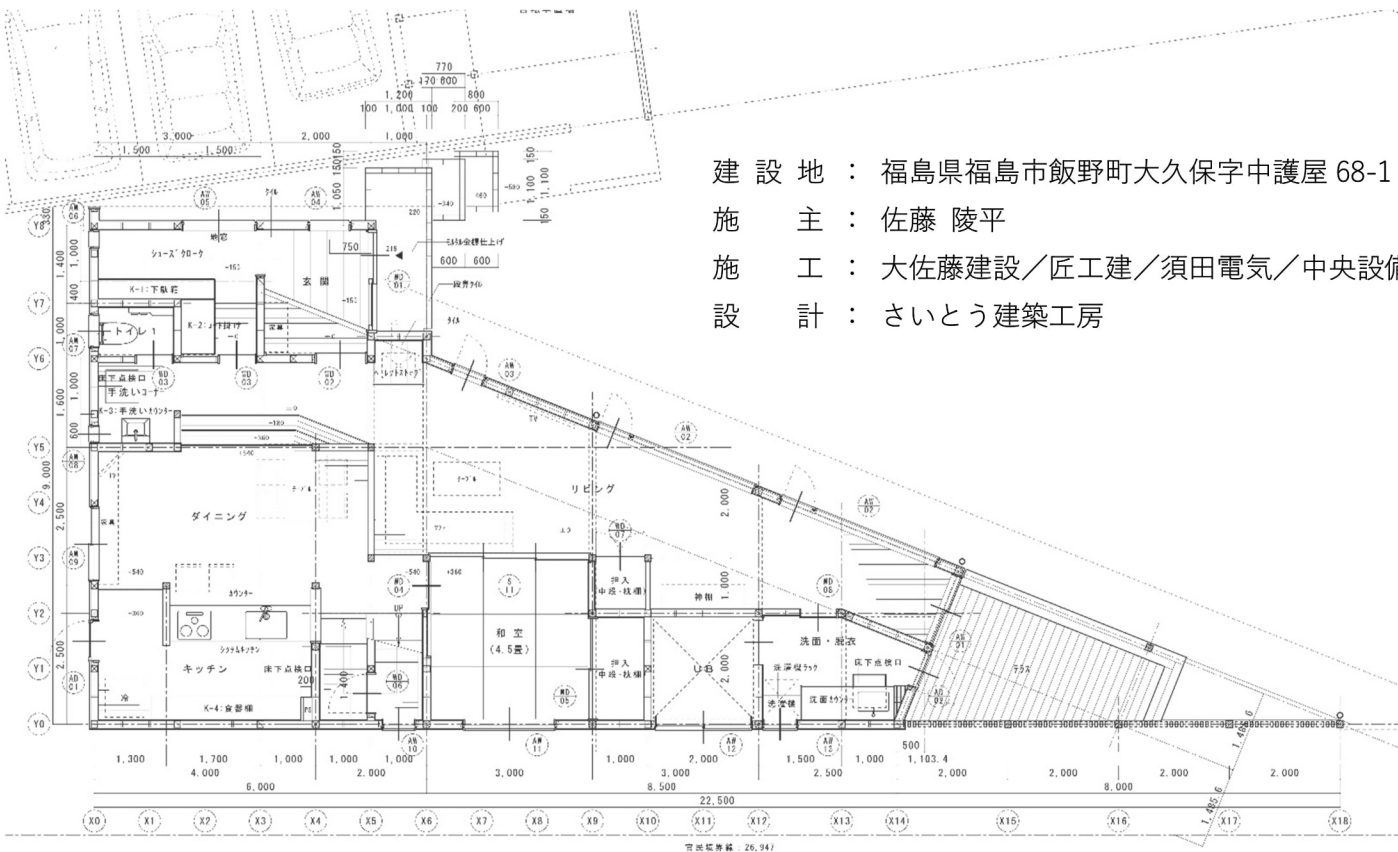
1階平面詳細図
